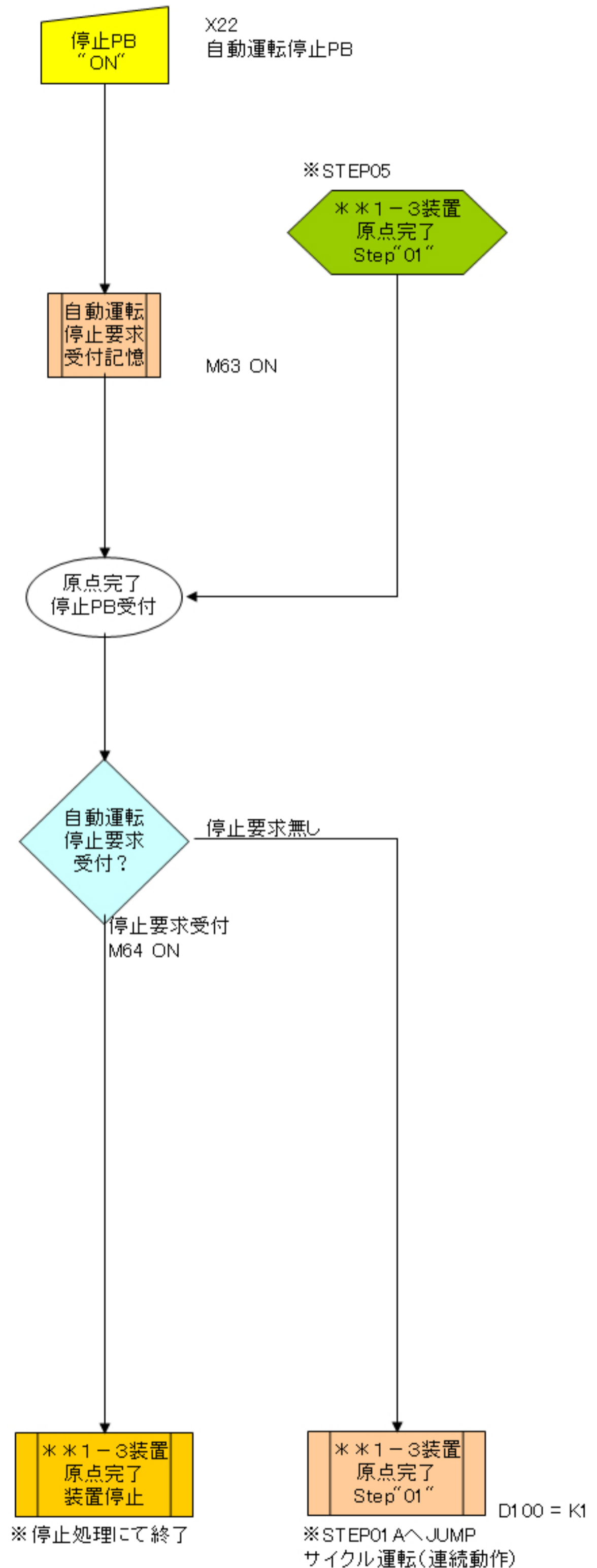
装置停止(1サイクル停止)
