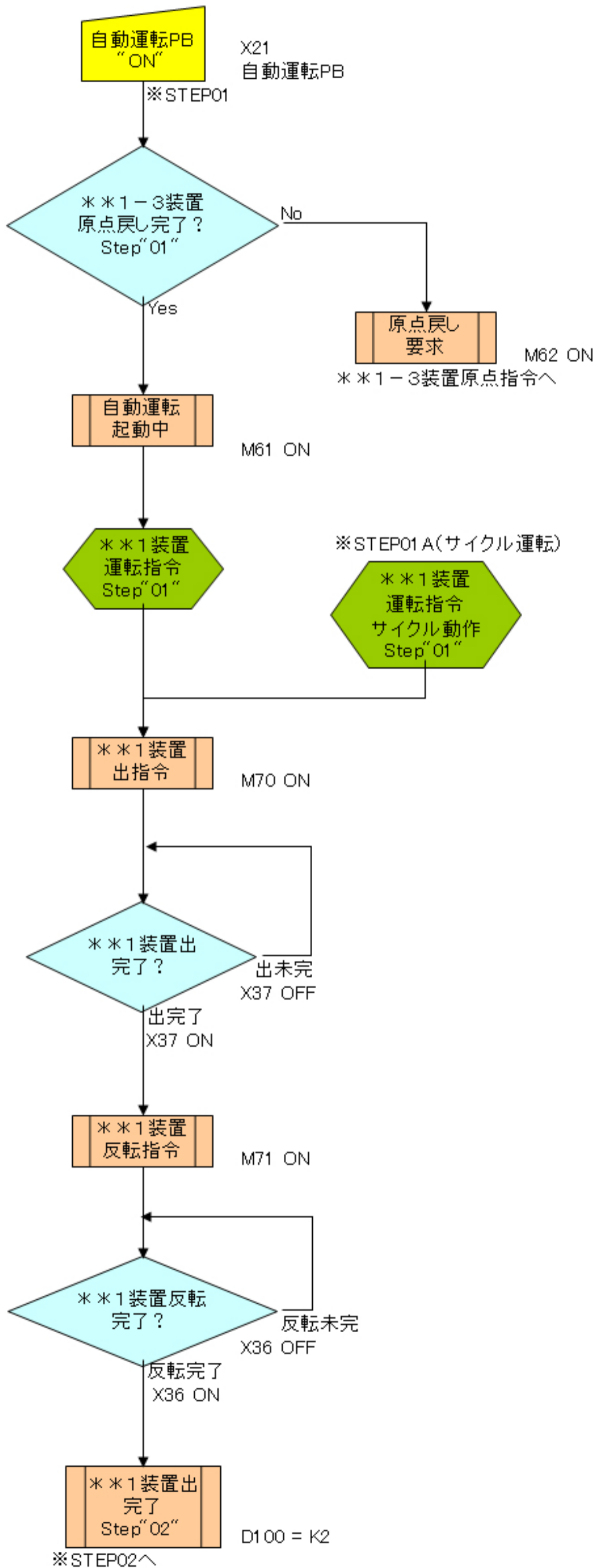
※※1装置動作&自動運転フロー図
